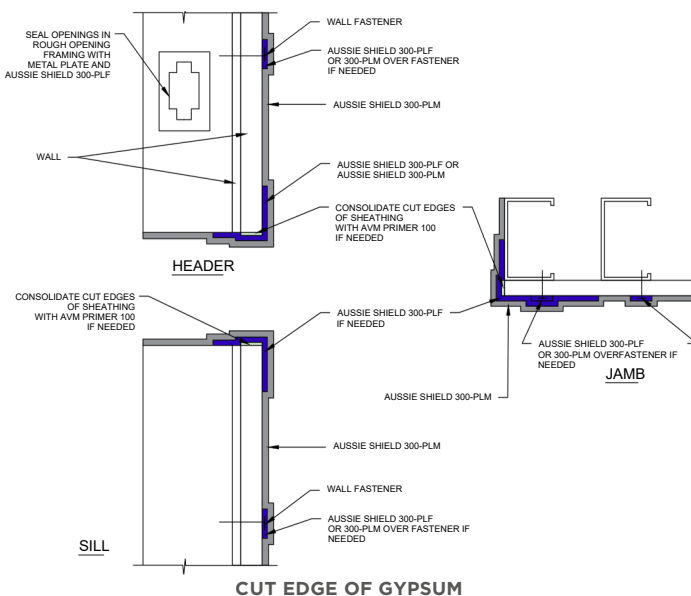
CUT EDGE OF GYPSUM
